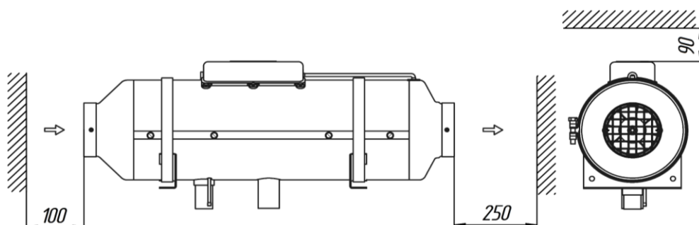
Abb. 1b - Abstand zu den Wänden
