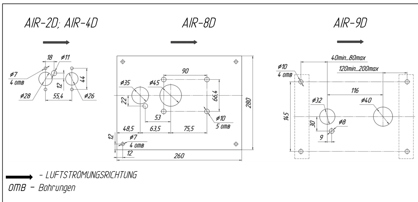
Abb. 3 - Befestigungsbohrungen
