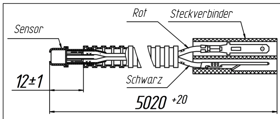
Abb. 23 - Temperatursensor
