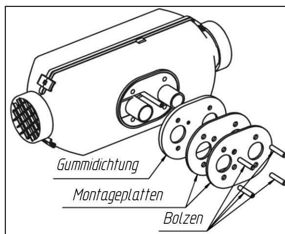
Abb. 2a - Montageplatten
