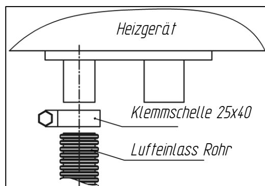
Abb. 4 - Anschluss der Luftleitung an das Heizgerät
