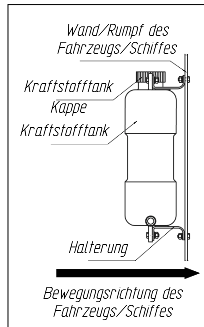
Abb. 16 Installation des Kraftstofftanks
