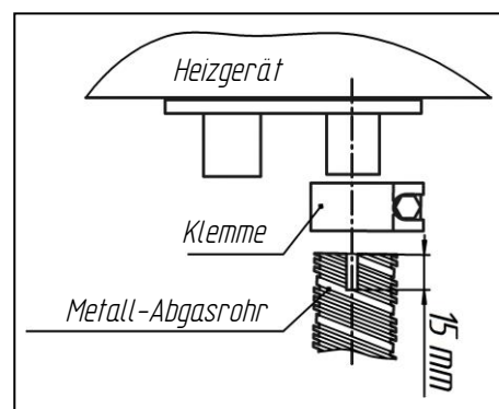
Abb. 8 - Befestigung des Metallrohrs am Heizgerät
