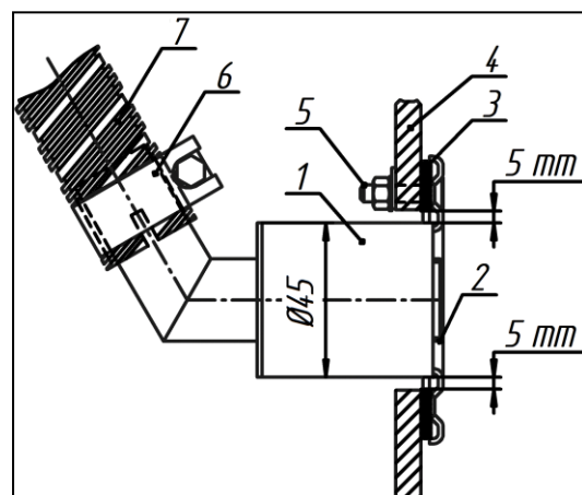
Abb. 13 - Montage des Auspuffrohres
