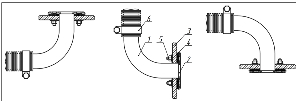
Abb. 7 - Montage des Luftansaugrohrs
