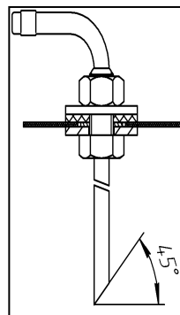
Abb. 15a - Installation des Kraftstoffsaugschlauches
