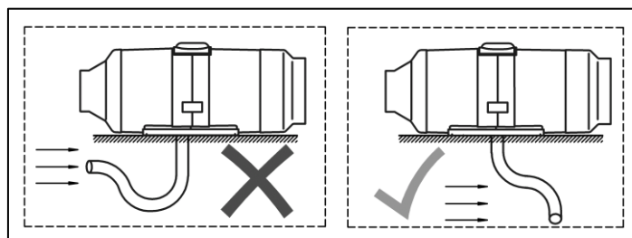
Abb. 5 - Position des Luftansaug-/Abgasrohrs
