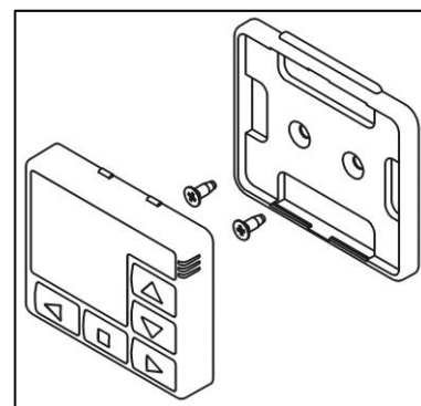
Abb. 24 – Montage des Bedienfeldes PU-27 mit einer Montagehalterung.
