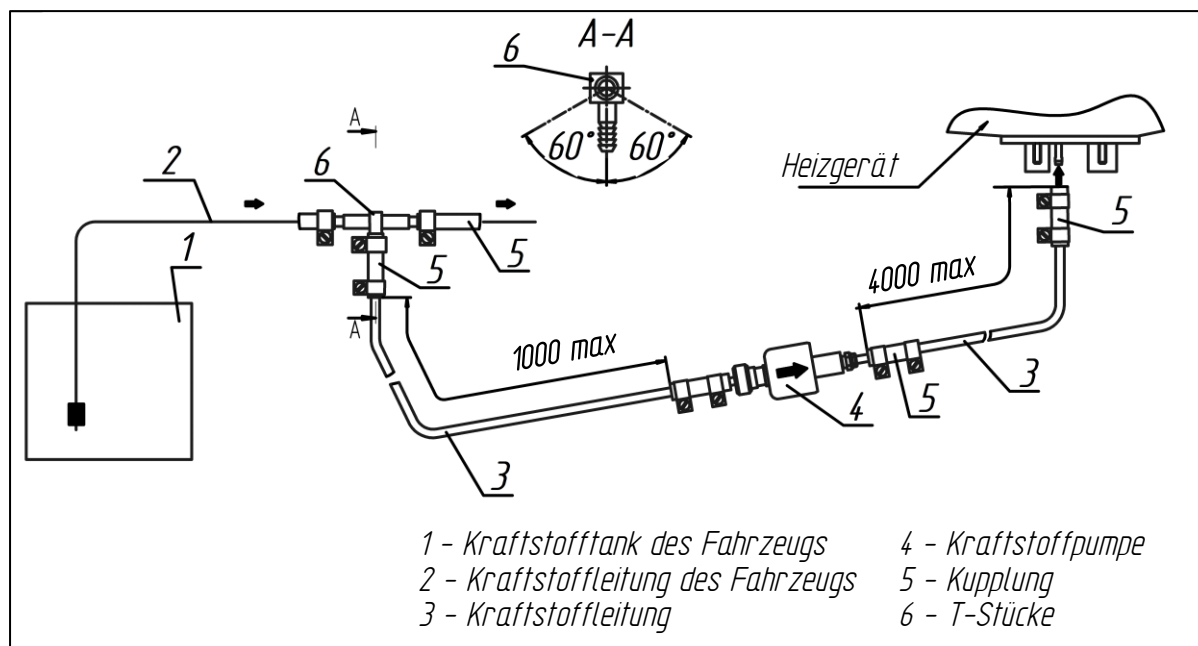
Abb. 17 - Kraftstoffansaugung mit einem T-Stück
