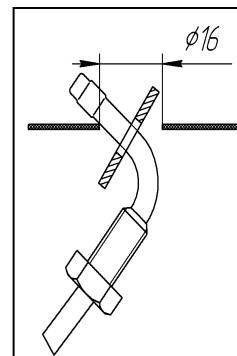
Abb. 15b - Installation der Unterlegscheibe.
