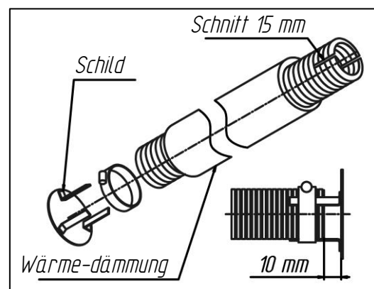
Abb. 9 - Auspuffrohrschild
