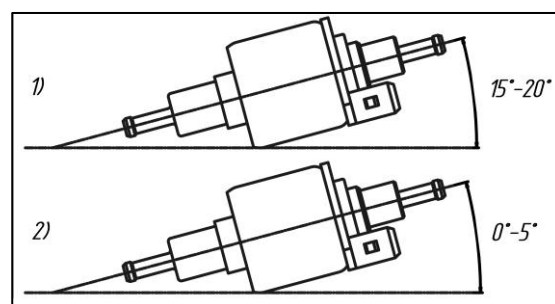
Abb. 18 - Installationswinkel der TH-9; TH-10; TH-11 Kraftstoffpumpe (1) und Thomas Magnete (2) Kraftstoffpumpe.
