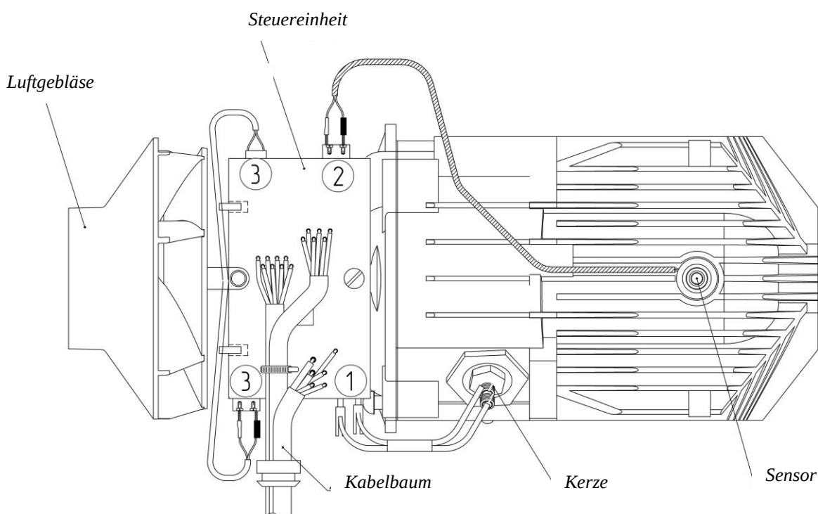
Abb.2 – Heizkörper.
