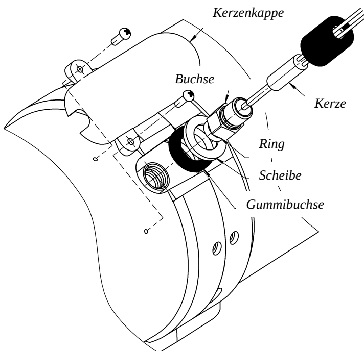
Abb. 4 - Kerze mit Montagesatz.
